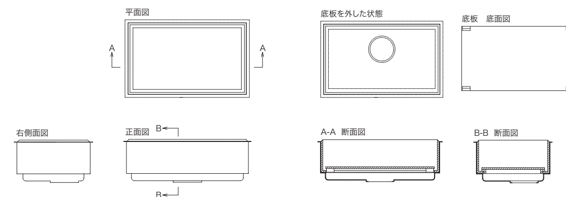
シンク詳細図 ※ネオリスを使用したシンクの一例です。
